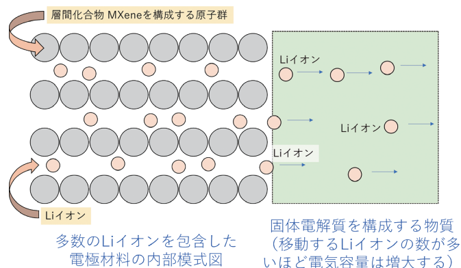
全固体電池用電極材料の構成図
