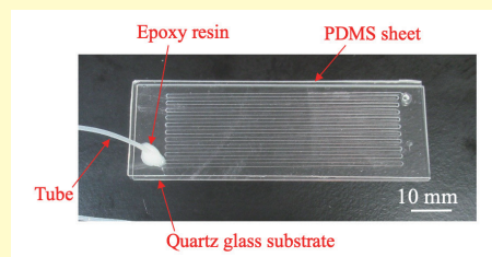
マイクロ流路デバイスの試作
