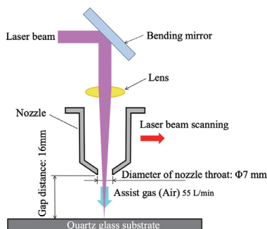
レーザによるマイクロ流路加工法
