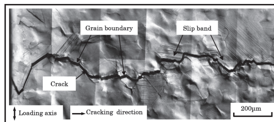
図3 溶体化処理したAZ61 合金での疲労き裂
