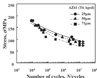
図2 T6 時効させたAZ61合金の疲労特性
