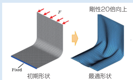
Fig. 1 薄板構造の最適設計の例
