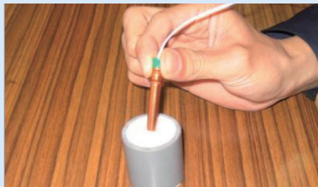
容器内の爆薬を起爆用の電気雷管で発破すると瞬時に加工・成形できる
